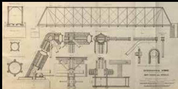
Most międzynarodowy między Erie a Buffalo, jedna z sekcji mostu. Gzowski, C. S., Toronto: Copp, Clark and Co., 1873.
